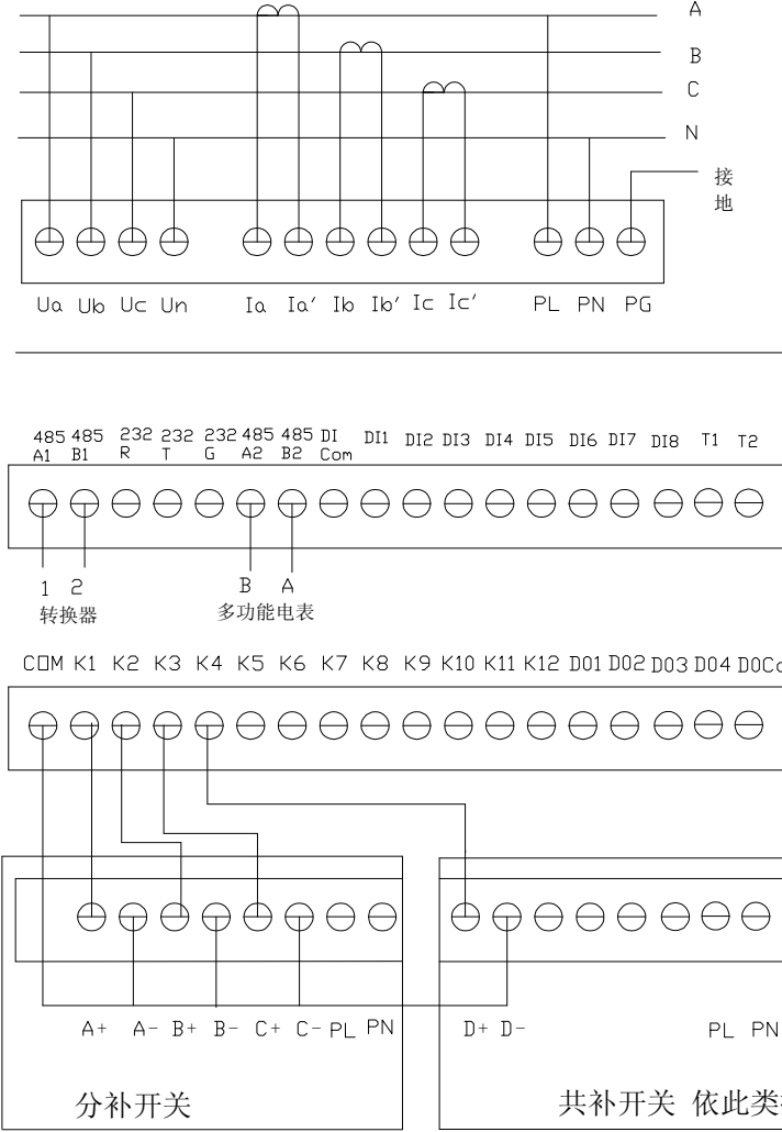
接线示意图
