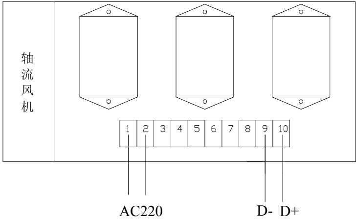
共补接线图
