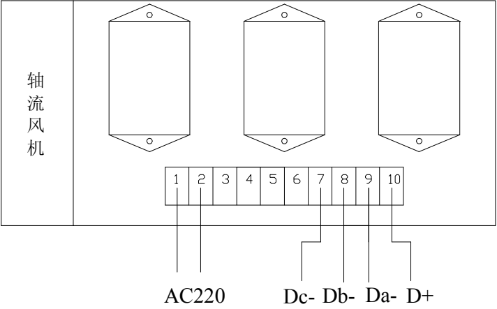
分补共负接线图
