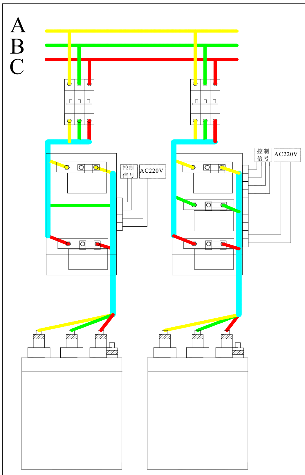
一次接线示意图
